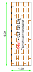
PIANEROTTOLO INTERNO - S=120 mm Superficie lorda (VxP) = 4,80 mq Lato inferiore faccia a vista
