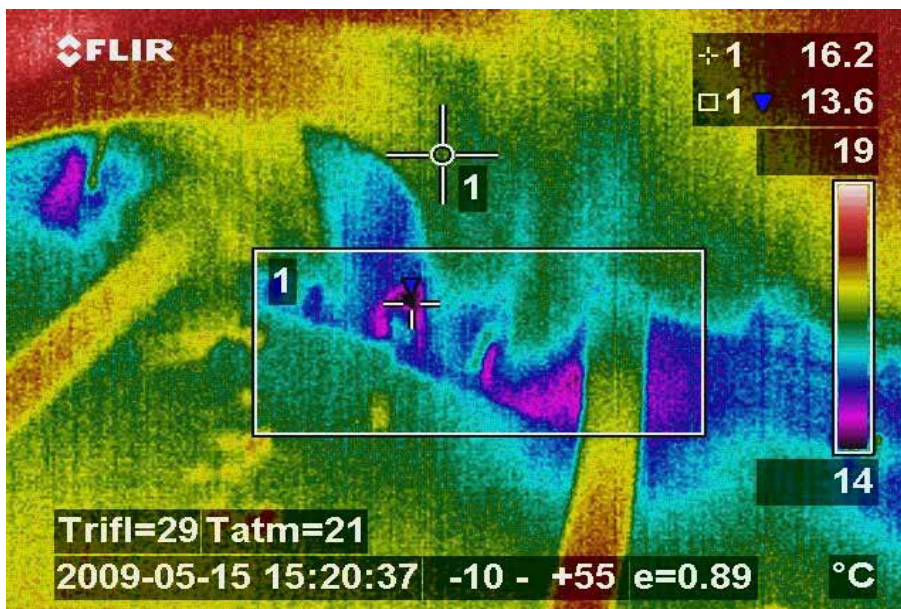
Individuazione perdite con termocamera
