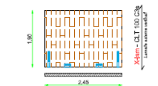
PARETE ESTERNA VANO TECNICO - S=100 mm Superficie lorda (VxP) = 4,65 mq
