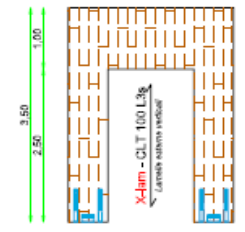
PARETE INTERNA MAGAZZINO - S=100 mm Superficie lorda (VxP) = 9,16 mq
