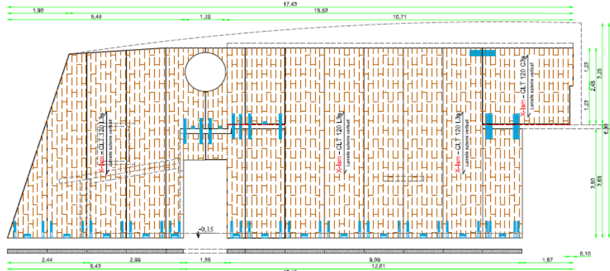
SVILUPPO LINEARE ELEMENTI X-LAM PARETE CURVA ESTERNA - S=120 mm Superficie lorda (VxP) = 95,85 mq - Lato interno faccia a vista
