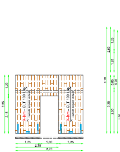
PARETE INTERNA VANO TECNICO - S=100 mm Superficie lorda (VxP) = 12,49 mq - Lato esterno faccia a vista
