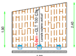
PARETE CONTRO MURO VANO TECNICO - S=100 mm Superficie lorda (VxP) = 6,00 mq
