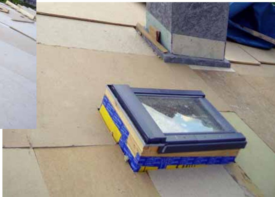
Tenuta al vento coperture in legno
